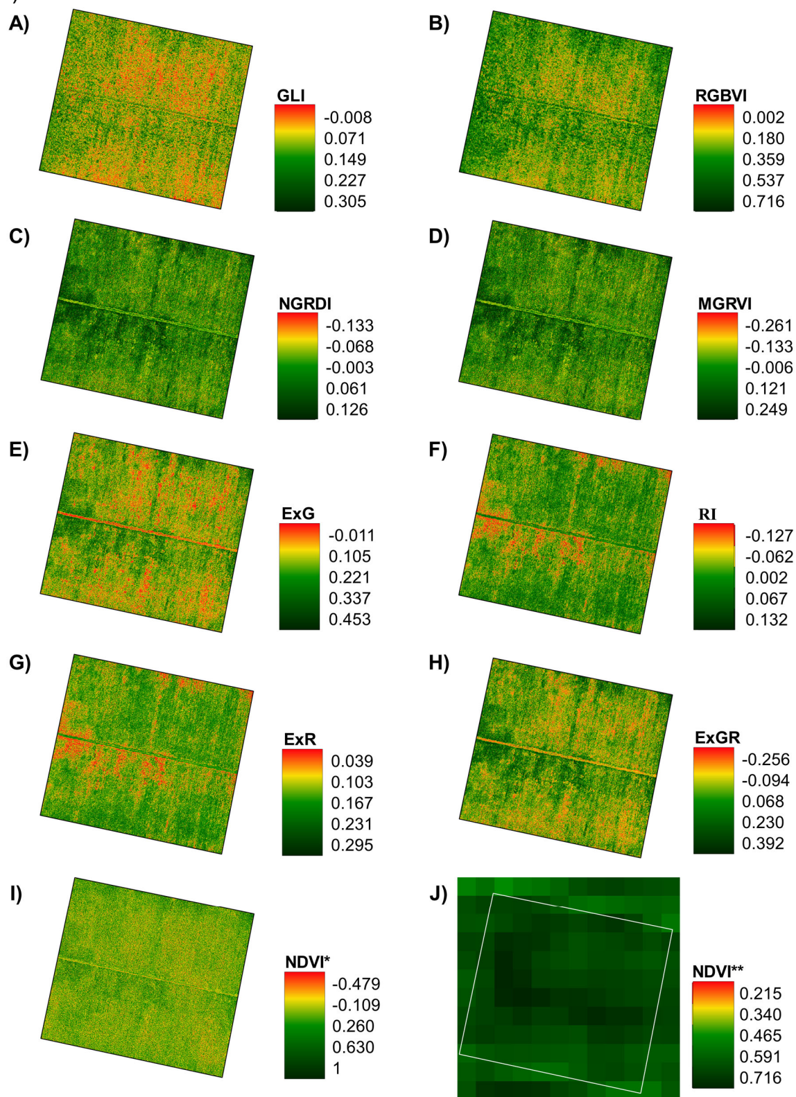
Figura 19. Índices de vegetação da área de cana-de-açúcar, em Juazeiro, Bahia, obtidos por imagem de VANT em 26/03/2021 (A, B, C, ..., I) e pela imagem Landsat 8 (J) em 17/03/2021.
