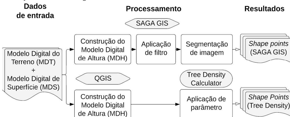
Figura 9. Etapas do processamento para geração do shape point por meio do Tree Density Calculator e Saga GIS.
