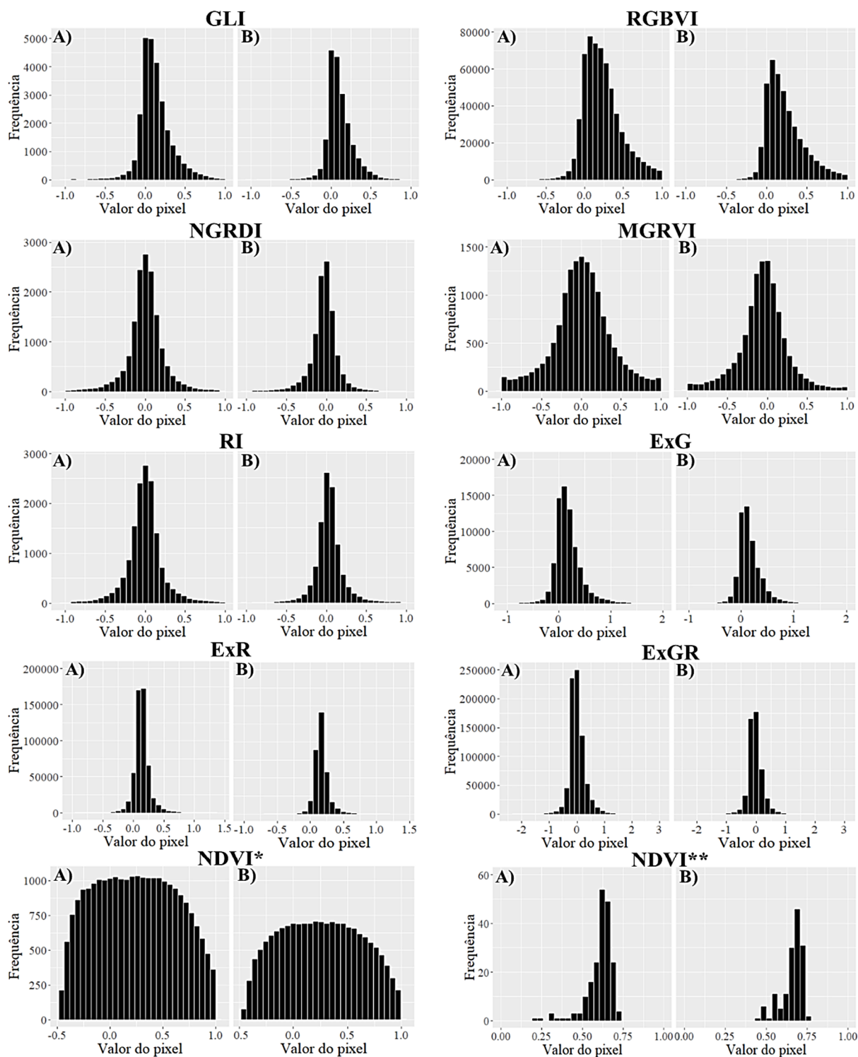
Figura 23. Histograma dos índices de vegetação obtidos em 26/03(A) e 18/06 de 2021(B), em área de cana-de-açúcar, em Juazeiro, Bahia.
