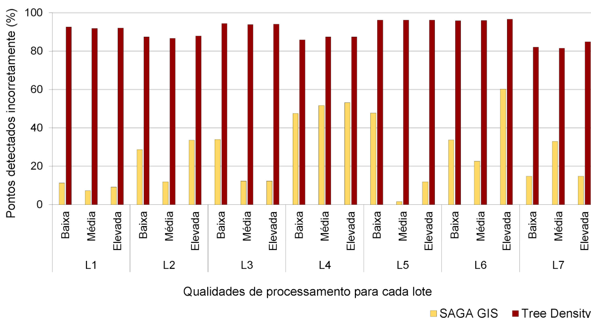
Figura 15. Percentuais de pontos detectados incorretamente para as áreas de manga (L1 à L6) e citrus (L7) para diferentes qualidades de processamento utilizando o SAGA GIS e o Tree Density Calculator .
