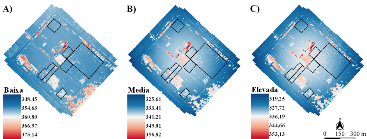
Figura 10. Modelos digitais de superfície obtidos a partir do processamento de imagens em qualidade baixa (A), média (B) e elevada (C).
