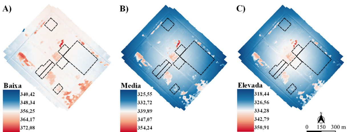
Figura 11. Modelos digitais do terreno obtidos a partir do processamento de imagens em qualidade baixa (A), média (B) e elevada (C).
