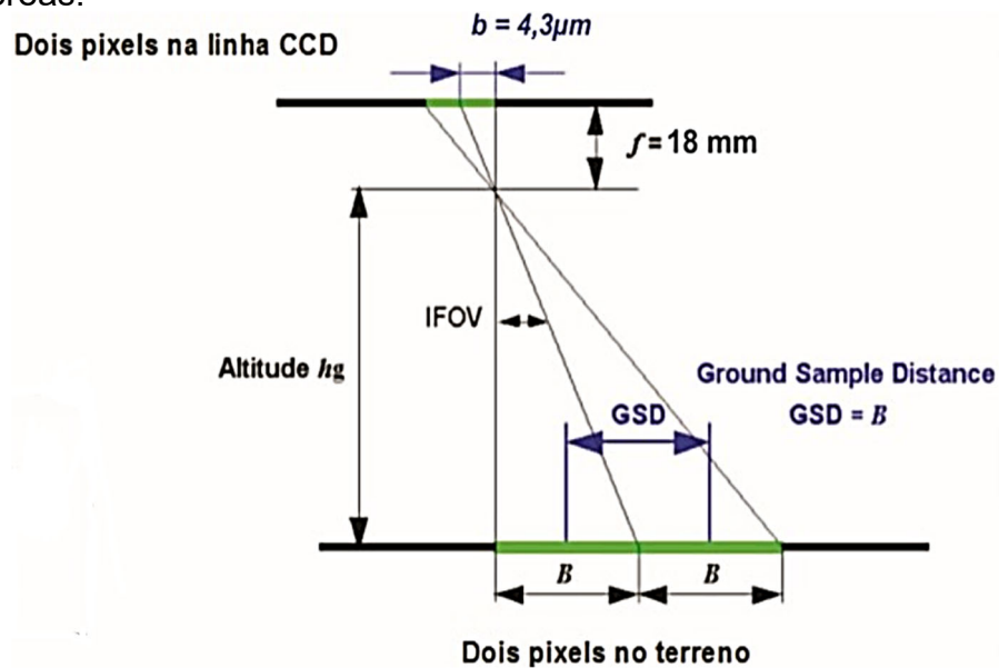
Figura 3. Parâmetros utilizados para cálculo do GSD ( Ground Sample Distance ) em imagens aéreas.
