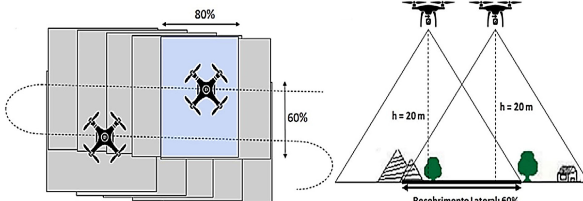
Figura 2. Esquema de cobertura aerofotogramétrica para tomada de imagens com região de sobreposição frontal (esquerda) e lateral (direita).
